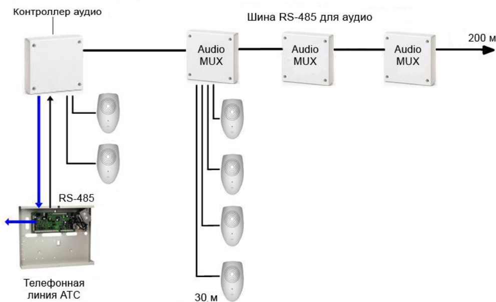
Рис. 1. Подсистема голосовой связи
